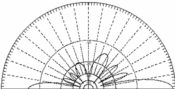
E-Plane
